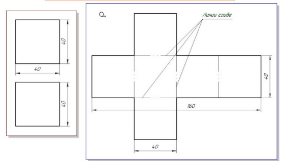
Построение чертежа развертки поверхностей куба
