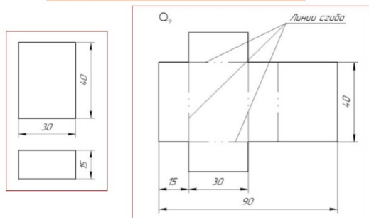
Построение чертежа развертки поверхностей прямоугольного параллелепипеда
