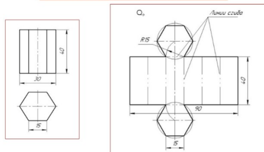
Построение чертежа развертки поверхностей шестиугольной призмы
